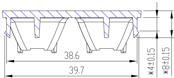
B-B 2:1
